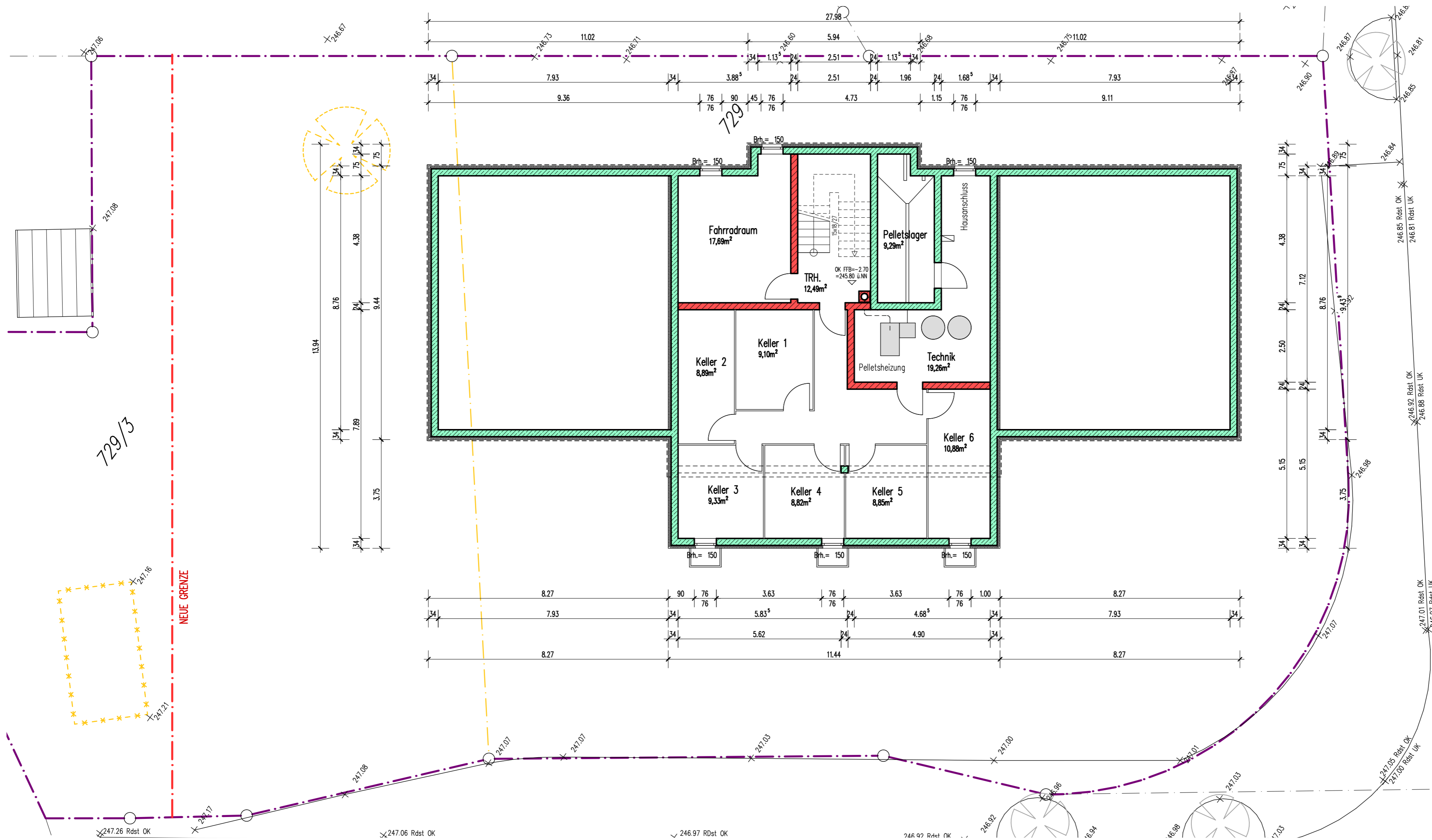
Grundriss Kellergeschoss
