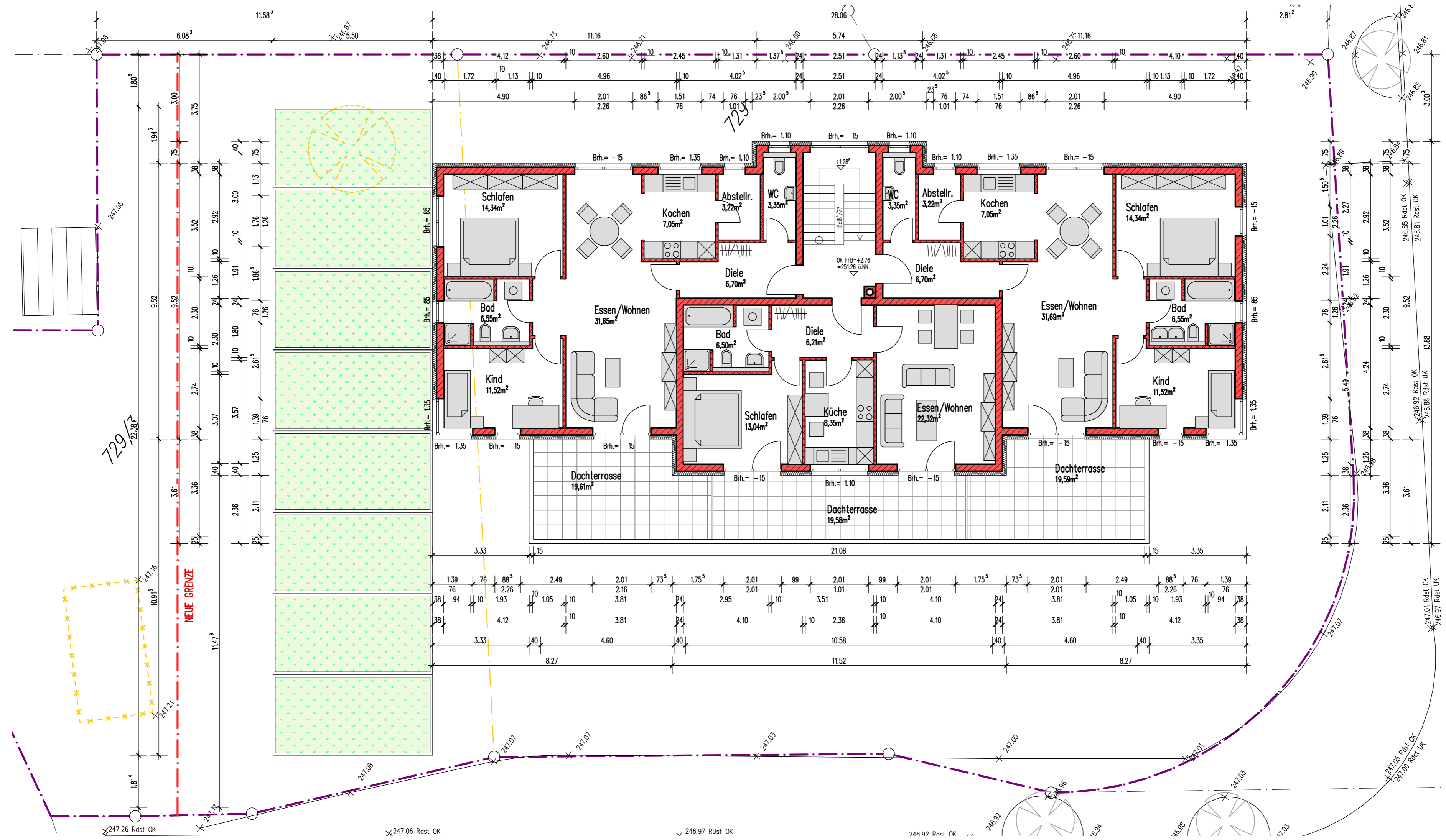
Grundriss Obergeschoss
